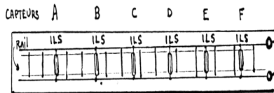
Banc de mesures
