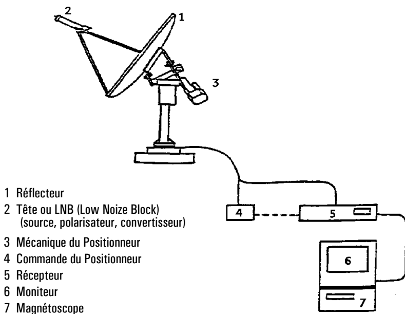
Figure 3 : Principaux constituants d'une station
