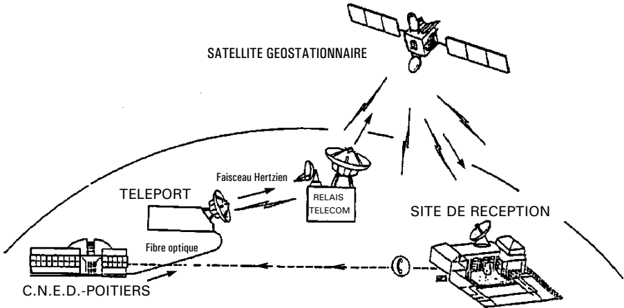
Figure 4 : Vidéotransmission interactive Circuit d'interactivité (schémas simplifiés)
