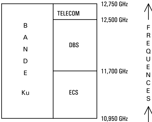
Figure 2 : Les bandes de fréquences les plus utilisées en télévision par satellite
