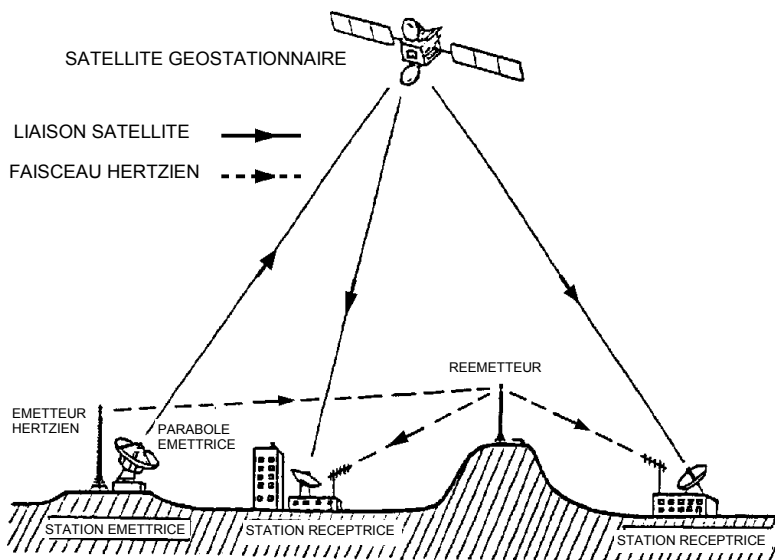
Figure 1: Transmission par faisceau hertzien et par satellite
